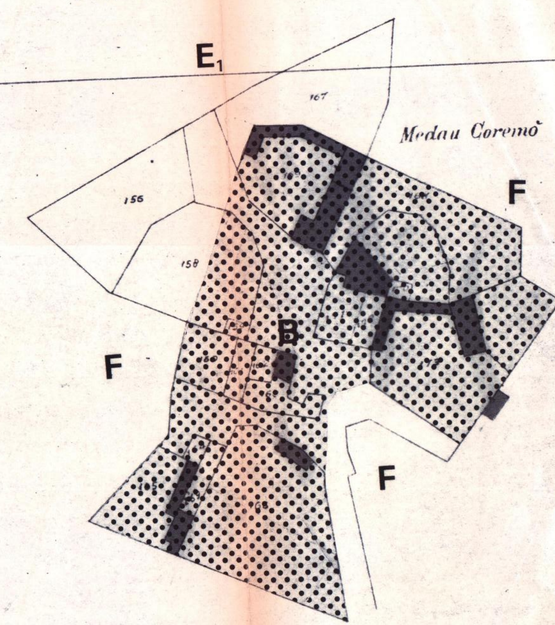
Sviluppo A Scala 1:1000
